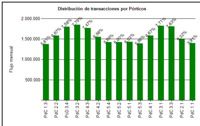
Gráfico 3: Distribución de Flujos por Pórtico de Cobro, Marzo 2015. Fuente: Reporte 29 SICE.
